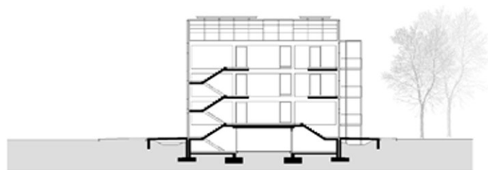
Querschnitt Treppenhaus
